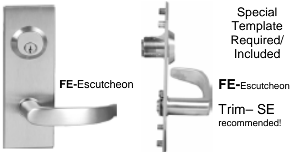
Escutcheon Dimensions 3/16" (D) x 2-5/8" (W) x 8" (L)
